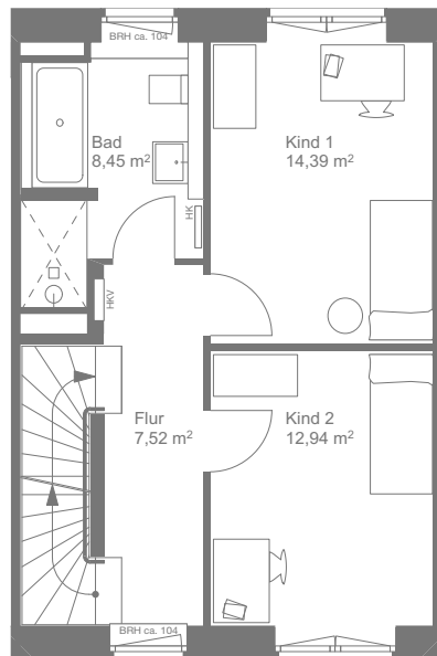
1. Obergeschoss
